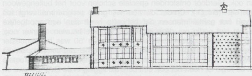
Definitief ontwerp gevelaanzicht VGLO-school Cuperstraat.
