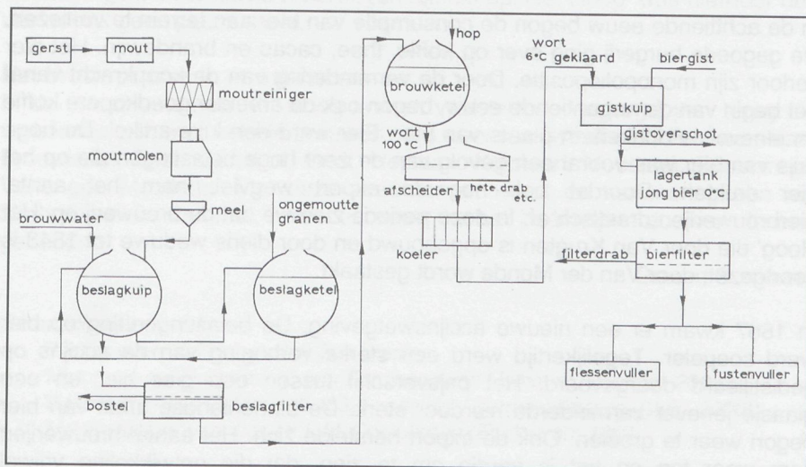
Schematische voorstelling van het brouwproces naar Het Bierboek door drs J.F.L.M. Cornelissen, pag. 122.
