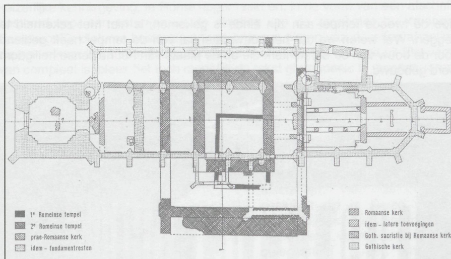
De opgravingsplattegrond uit 1947 geeft inzicht in de verschillende bouwstadia.
