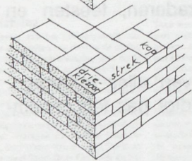
Vlaams verband massief
