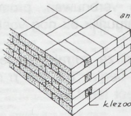
Vlaams verband massief
