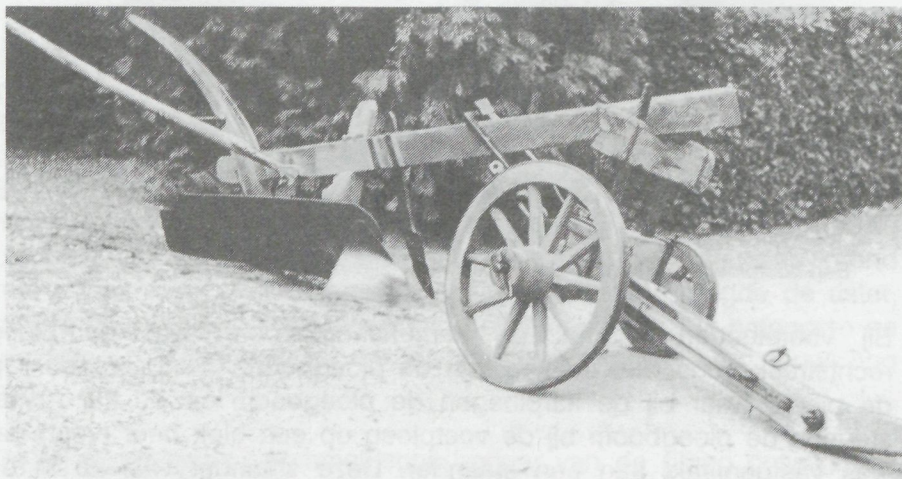
Foto van een Betuwse karploeg, met een ploegspade die als tweede staart diende.
