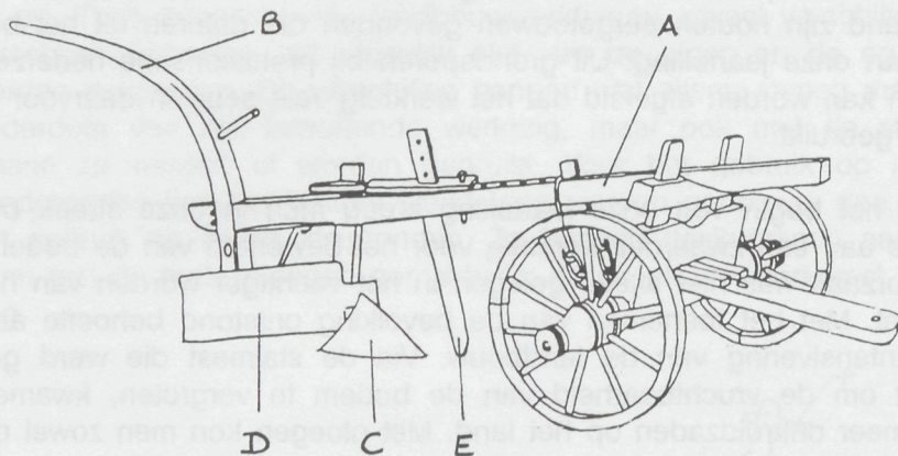
Tekening van een karploeg: A=ploegboom, B=staart, C=schaar, D=rister en E=kouter. De ploeg is bevestigd op een kar met een groot en een klein wiel.
